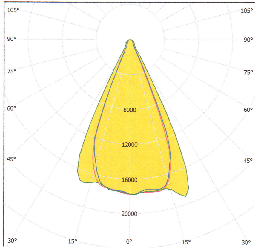
Рисунок 1 – КСС образца светильник светодиодный TL-PROM 100 PR PLUS (К) в поперечной (С0-С180) (красная кривая), продольной (С90-С270) (синяя кривая) и в плоскости максимальной силы света (С44-С224) (зеленая кривая)
