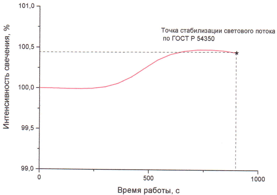
Рисунок 2 – График стабилизации светового потока образца светильник светодиодный TL-PROM 100 PR PLUS (К)
